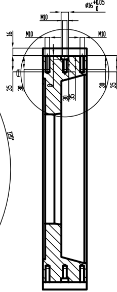
KESİT C-C
