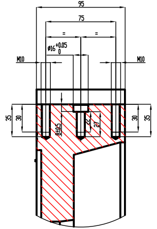
DETAY D BÜYÜKÇEK 1 : 2
