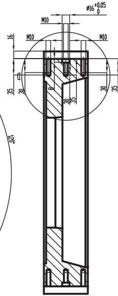
KESİT C-C
