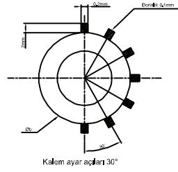
B-BAKIŞI
