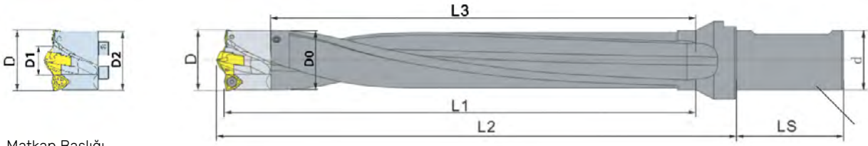
Matkap Başlığı Drill Head
