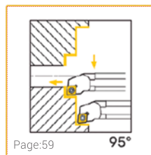
S...SVJBR/L
