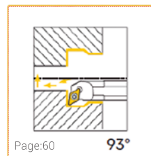
S...SVUBR/L
