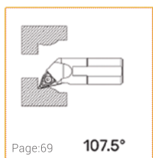
S...MTQNR/L
