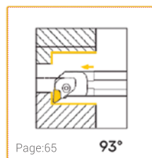
S...MTUNR/L
